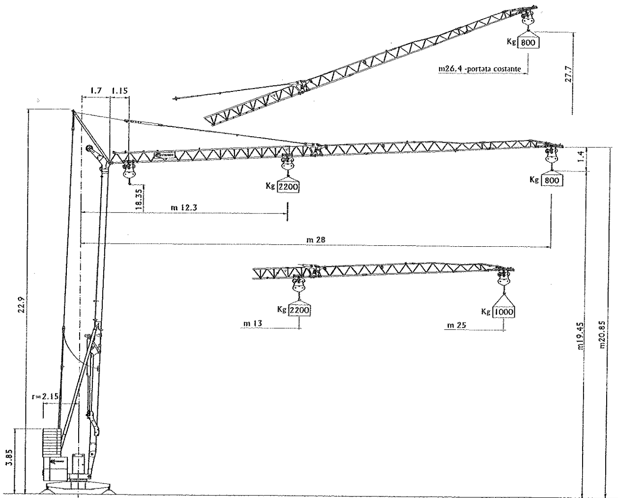
TAVOLA 1: CONFIGURAZIONI DELLA GRU CON BRACCIO DA m - 28 - 25 ORIZZONTALE O IMPENNATO
