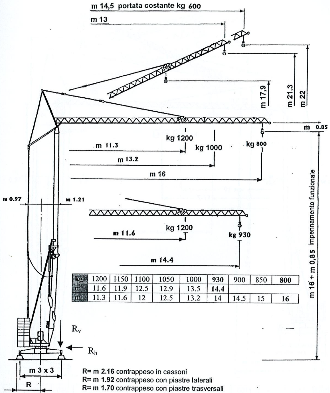
TAVOLA 1: CONFIGURAZIONI DELLA GRU CON BRACCIO DA m - 14,44 - 16 ORIZZONTALE O IMPENNATO
